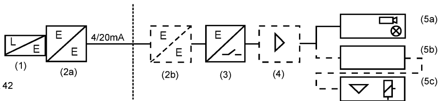
Schema der Überfüllsicherung für alle Typen und eingebautem Messumformer FEL60H
