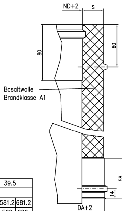
Elementverbindung
