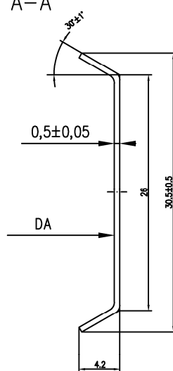
Schnitt A-A
