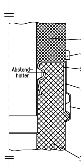
Elementverbindung
