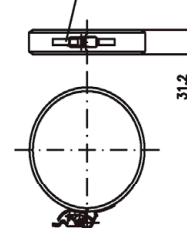
Spannschelle ND150-ND600 Verschraubung
