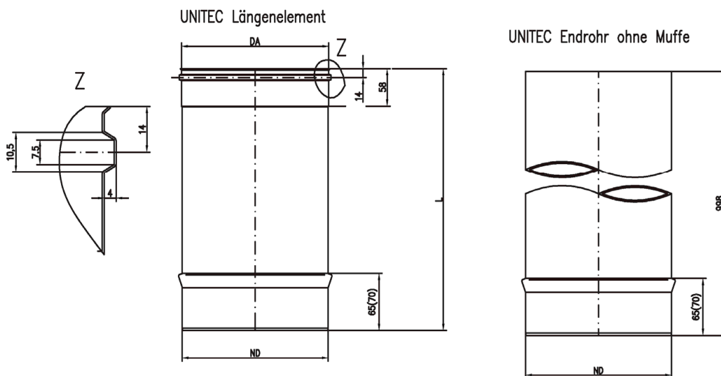
UNITEC Muffen- / Steckverbindung
