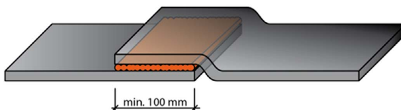
Abbildung 1: Verklebung des Stoßes mittels "gelbrot EPDM-Folienkleber"
