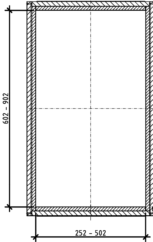
Schnitt C-C
