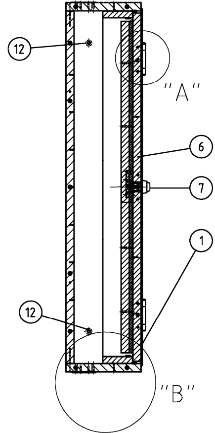
Schnitt B-B
