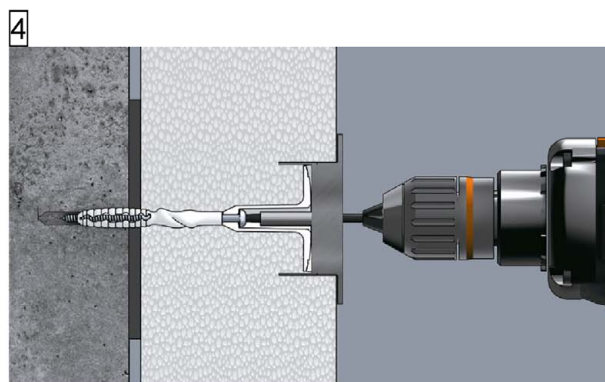
vertiefte Montage mit STR-tool
