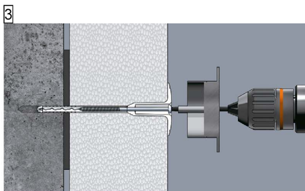
vertiefte Montage mit STR-tool
