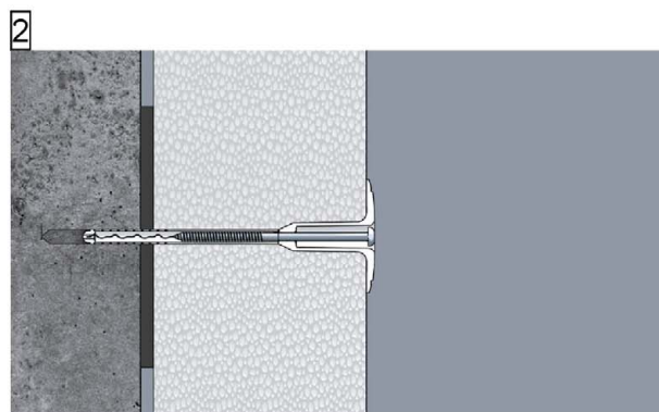
2 Dübel einsetzen
