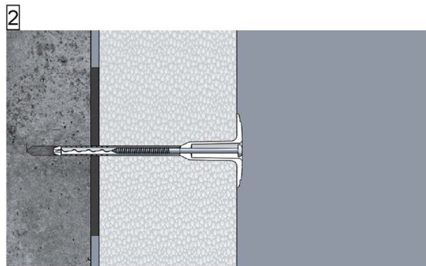
Dübel einsetzen
