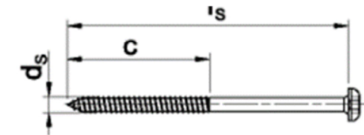
Markierung der Verankerungstiefe
