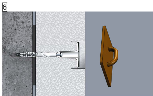
ejotherm STR-Rondelle einsetzen und mit einem Reibebrett oberflächenbündig eindrücken
