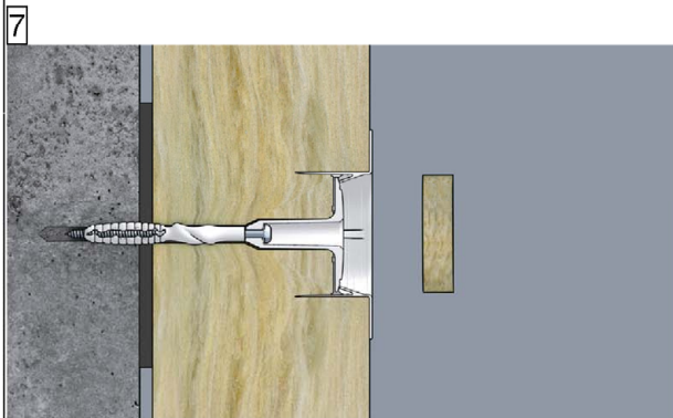
Insert the ejotherm STR-Cap
