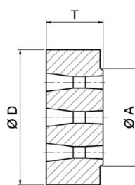
Lochscheibe
