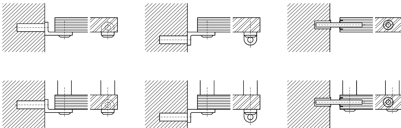
Wandanker: Winkel
