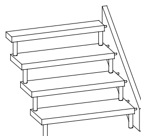
WF2 (2 Wandanker)
