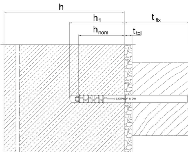
Bild 1: Einbauzustand: Kopfform: Senkkopf
