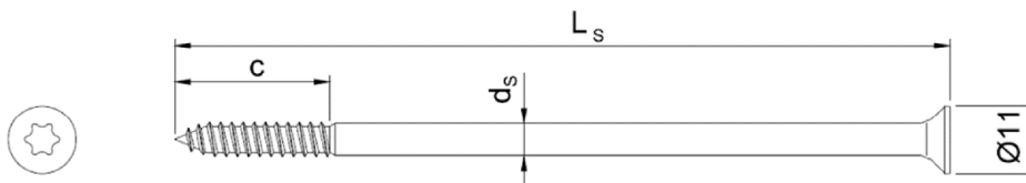
Bild 1: Dübeltyp Senkkopf (S)
