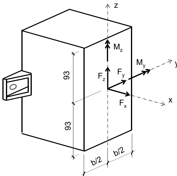
Abbildung C2: Darstellung der Schnittgrößen für die Bauteilwiderstände F_x , F_y , F_z , M_y und M_z an der Druckverteilerplatte der Schwerlastkonsole SLK-ALU-TTR und SLK-ALU-TTQ
