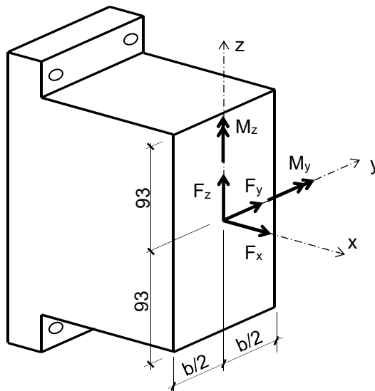
Abbildung C1: Darstellung der Schnittgrößen für die Bauteilwiderstände F_x , F_y , F_z , M_y und M_z an der Druckverteilerplatte der Schwerlastkonsole SLK-ALU-TR und SLK-ALU-TQ
