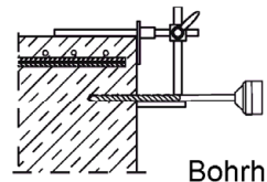
Bohrhilfe
