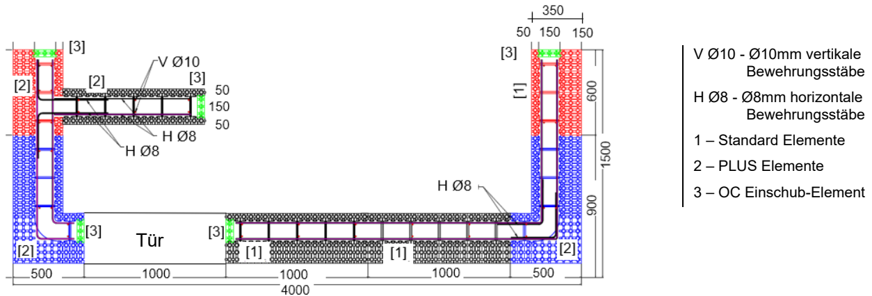
Abbildung 1: Skizze der ersten Lage der Versuchsstruktur
