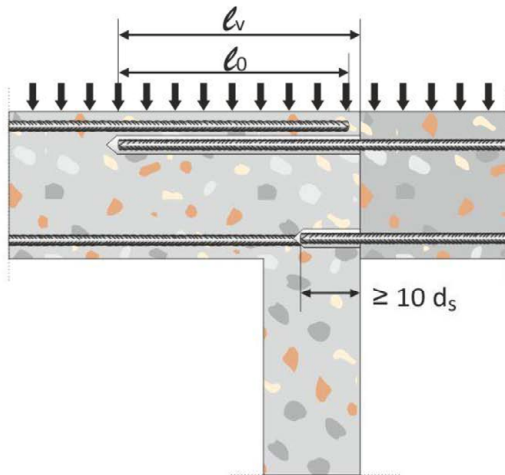
Bild A3: Endverankerung von Platten oder Balken (z.B. gelenkig gelagert bemessen)
