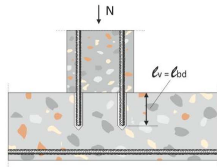
Bild A4: Bewehrungsanschlüsse überwiegend auf Druck beanspruchter Bauteile; Bewehrungsstäbe auf Druck beansprucht
