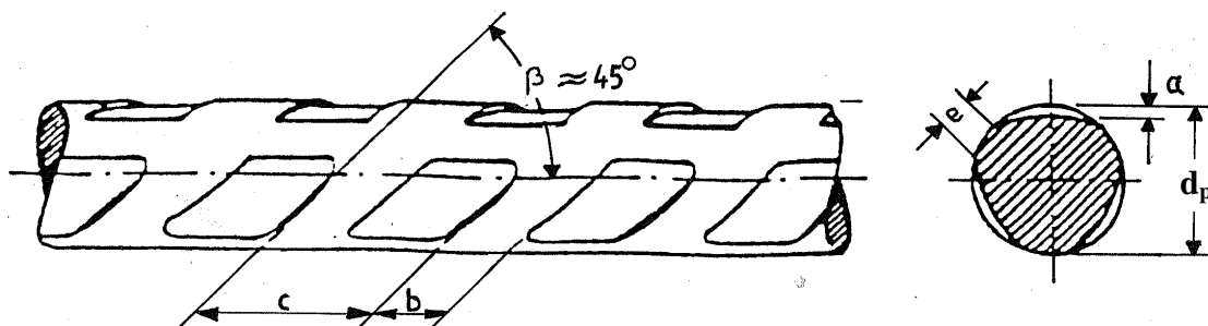
Bild 1: Ansicht des profilierten Spannstahldrahts
