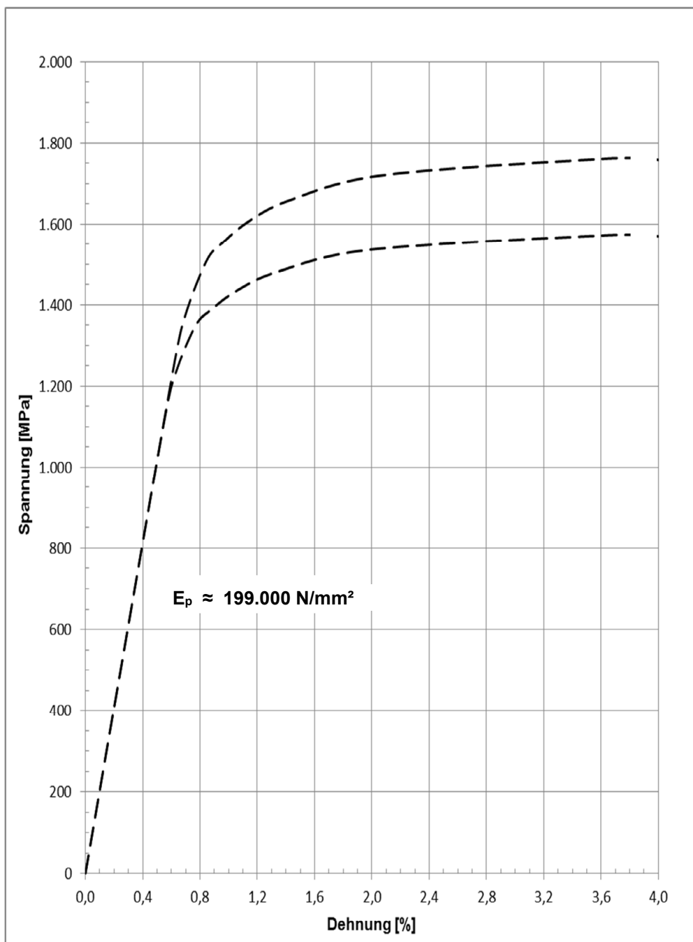
Bild 2: Prinzipieller Spannung-Dehnungs-Verlauf
