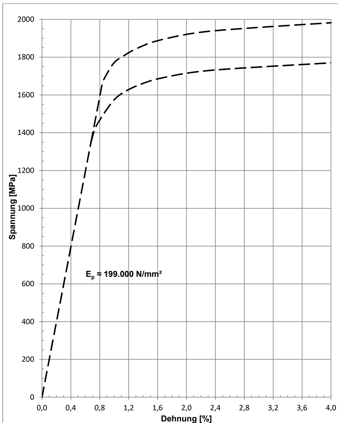
Bild 2: Prinzipieller Spannung-Dehnungs-Linie-Verlauf
