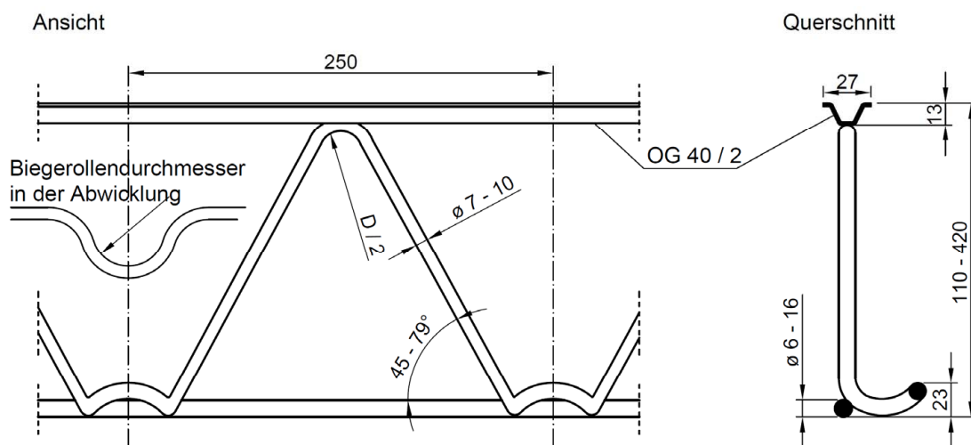
Bild 1: FILIGRAN - SE-Träger
