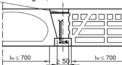
Bild 6: Rippendecke nach Anlage 8, Abschnitt 5
