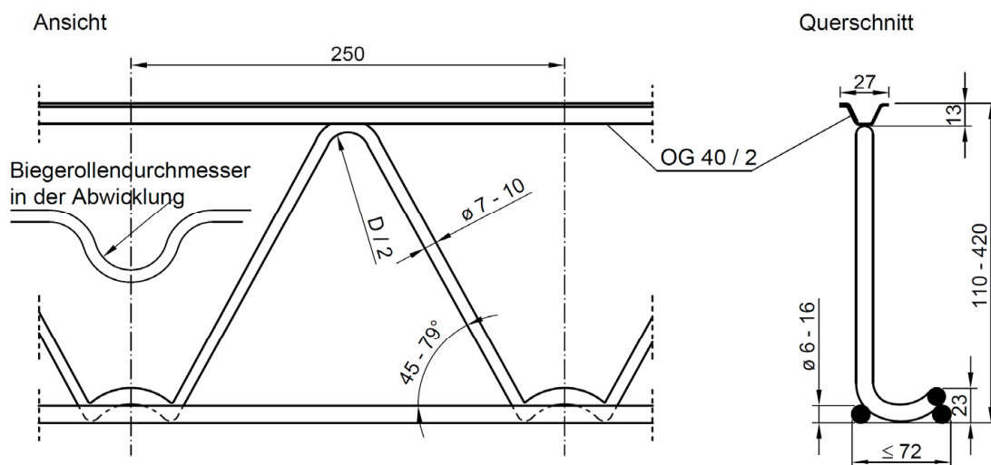
Bild 2: FILIGRAN - S-Träger
