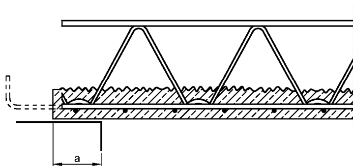
Bild 15: Auflagerung mit Montageunterstützung am Rand
