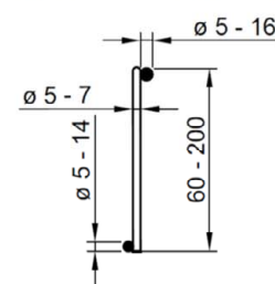
Bild 3: DH-Gitterträger
