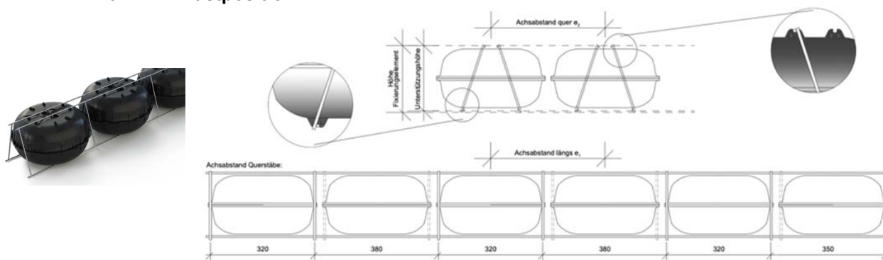
Bild 3: Darstellung Hohlkörper / Eco-Bewehrungsleiter (Eco-Fixierungselement) 10mm Einrastposition
