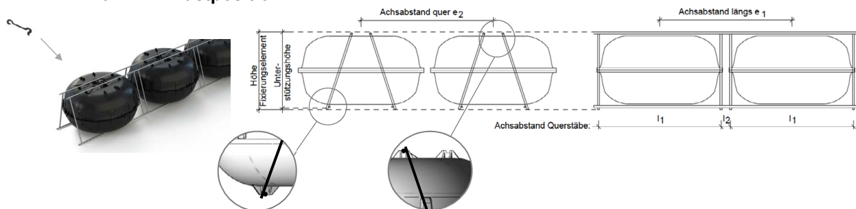
Bild 1: Darstellung Hohlkörper / Standard-Bewehrungsleiter (Standard - Fixierungselement) 10mm Einrastposition
