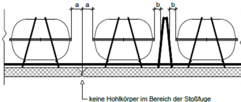
Bild 6: Mindestabstände der Cobiax Slim-Line-Einbauelemente
