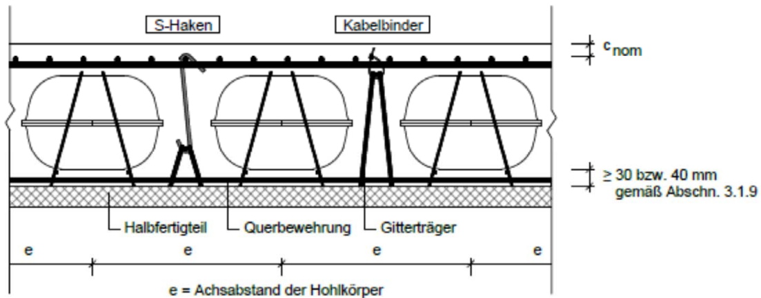
Bild 5: Lage der Cobiax Slim-Line-Einbauelemente auf den Halbfertigteilplatten und Auftriebssicherung mittels S-Haken oder Kabelbinder
