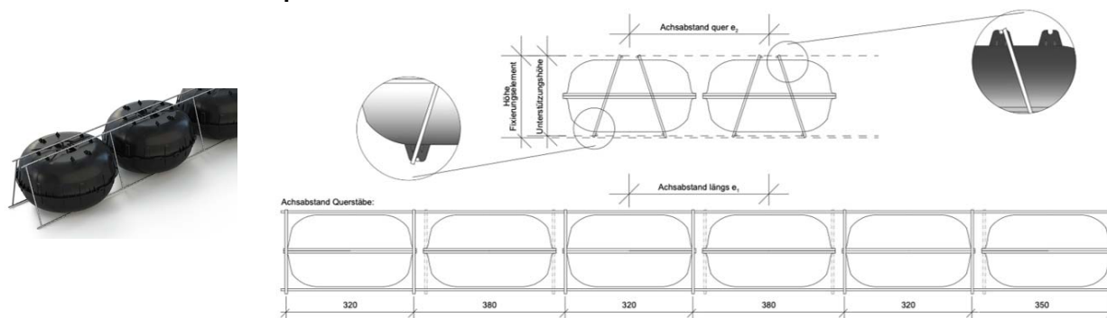
Bild 4: Darstellung Hohlkörper / Eco-Bewehrungsleiter (Eco-Fixierungselement) 15mm Einrastposition
