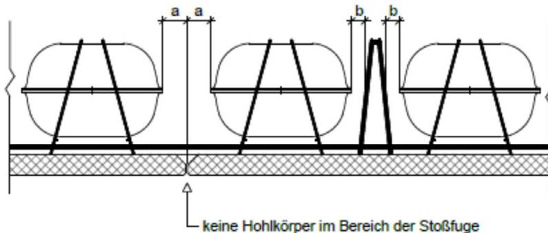
Bild 3: Mindestabstände der Cobiax Slim-Line-Einbauelemente
