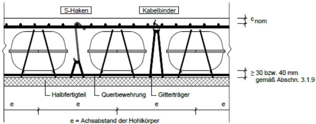
Bild 2: Lage der Cobiax Slim-Line-Einbauelemente auf den Halbfertigteilplatten und Auftriebssicherung mittels S-Haken oder Kabelbinder
