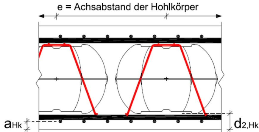
Bild 1: Querschnitt Hohlkörperdecke System "Cobias Slim-Line"
