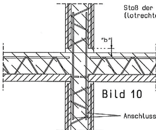
bewehrte Wände
