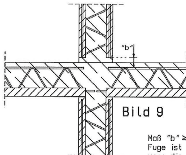
unbewehrte Wände
