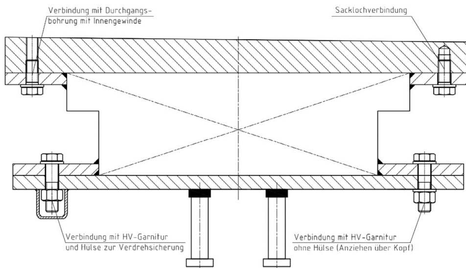
Bild 1: Einbausituationen
