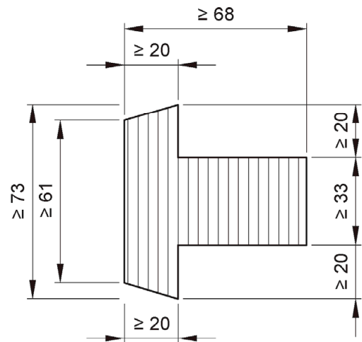
A-A
