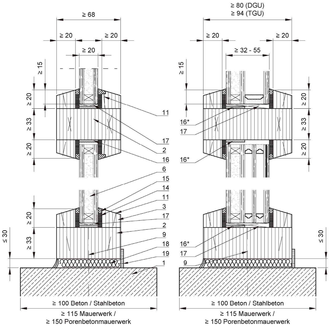
Ausführungsbeispiel mit Verbundglas
