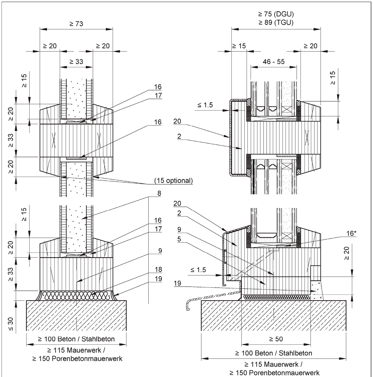
Schnitt D-D, E-E: Ausführung mit Ausfüllung
