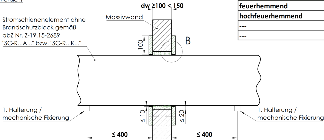
Schnittansicht
