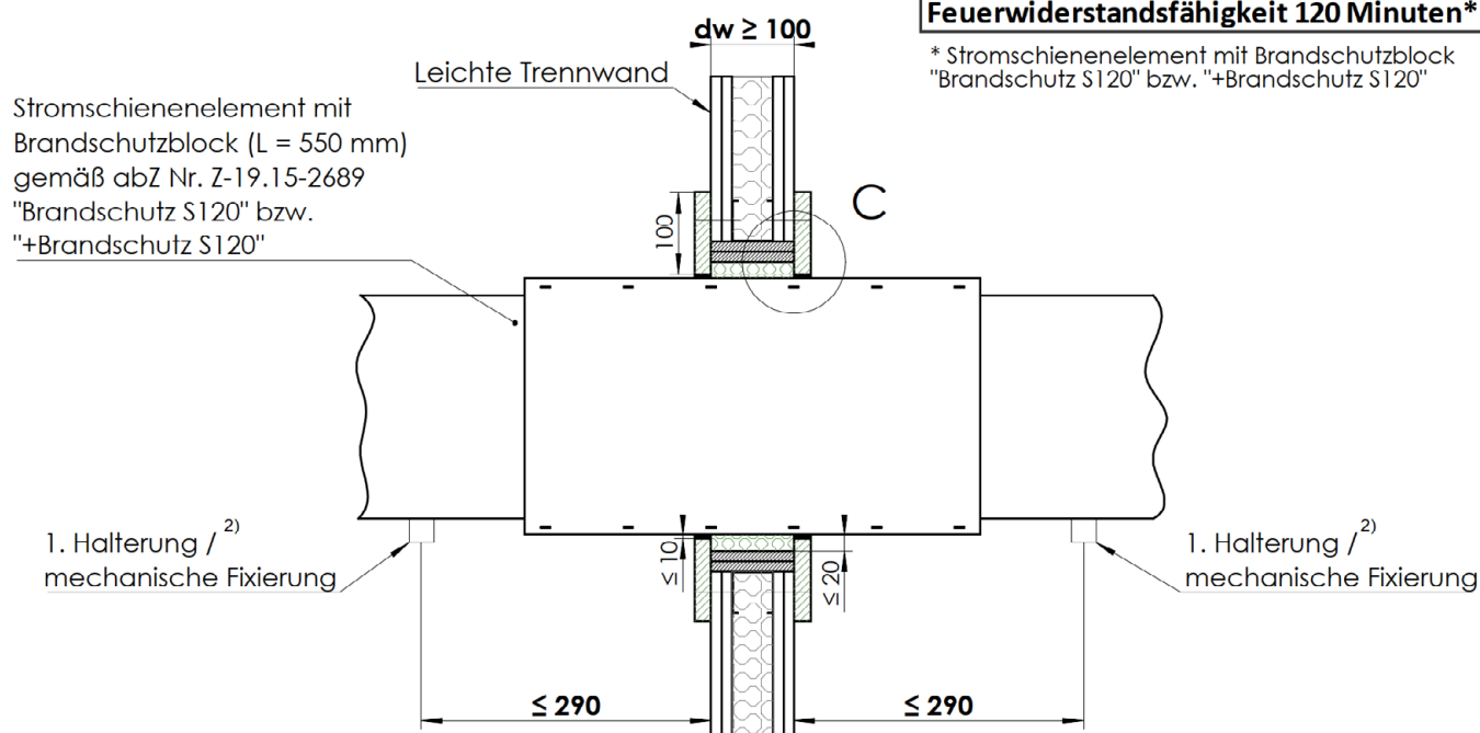
Schnittansicht
