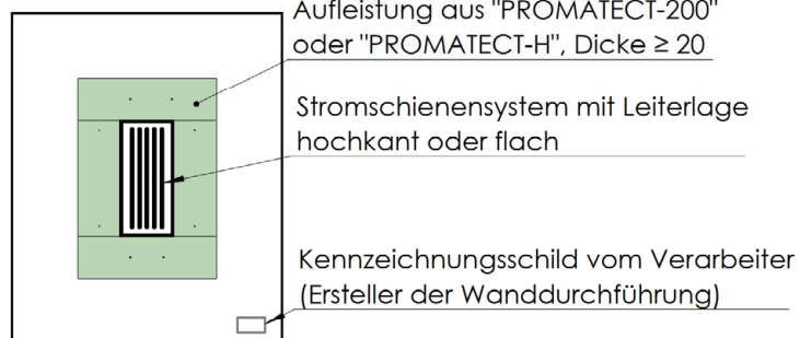
Frontansicht
