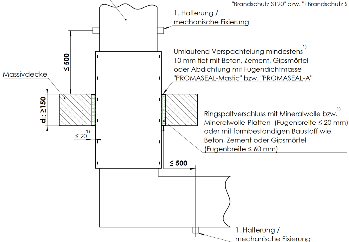
Einbau der Stromschienenelemente mit Brandschutzblock in der Rohbauöffnung
