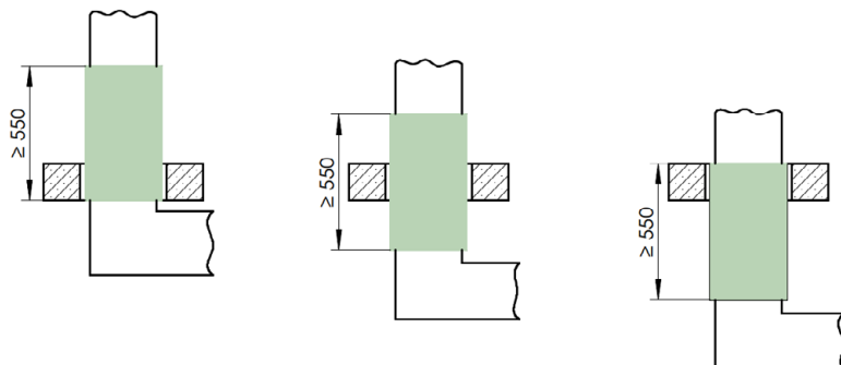
Einbau der Stromschienenelemente mit Brandschutzblock in der Rohbauöffnung
