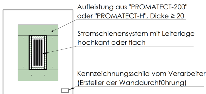
Frontansicht
