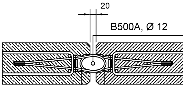
Bild 5: Regelfall Fuge horizontale Sollage
