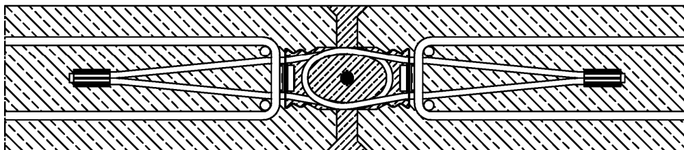
Bild 10: Wand - Wandverbindung
