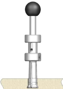
HVL-T (Hinterschnitt-Mindestvolumenlehre)
