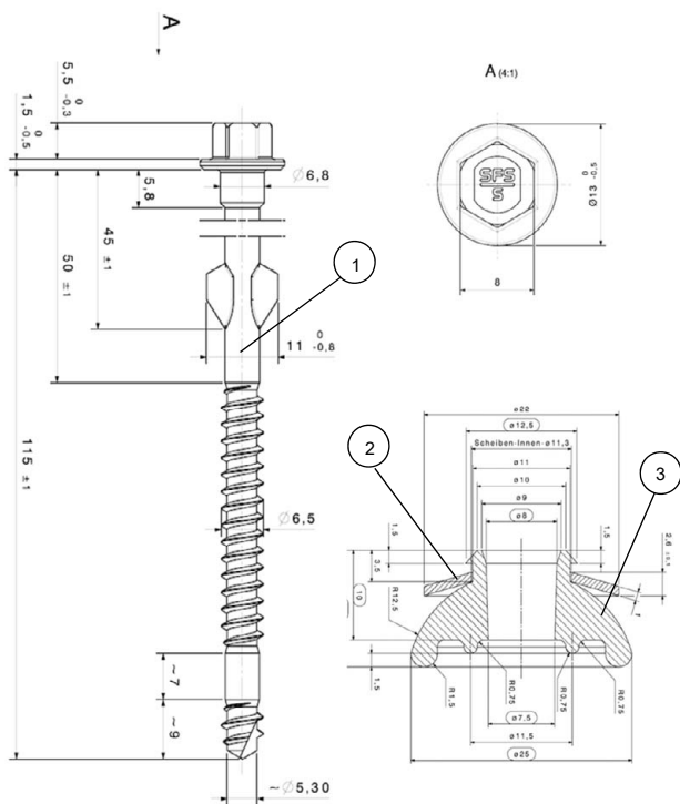
Bild 8: SFS SCFW-S-C11 6,5 x 115 mm
