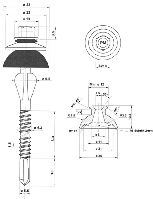
Bild 13: PMJ TOPEX Piasta 7442 6,5 x 115 mm
