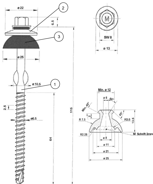
Bild 3: PMJ 745765115Z22 6,5 x 115 mm
