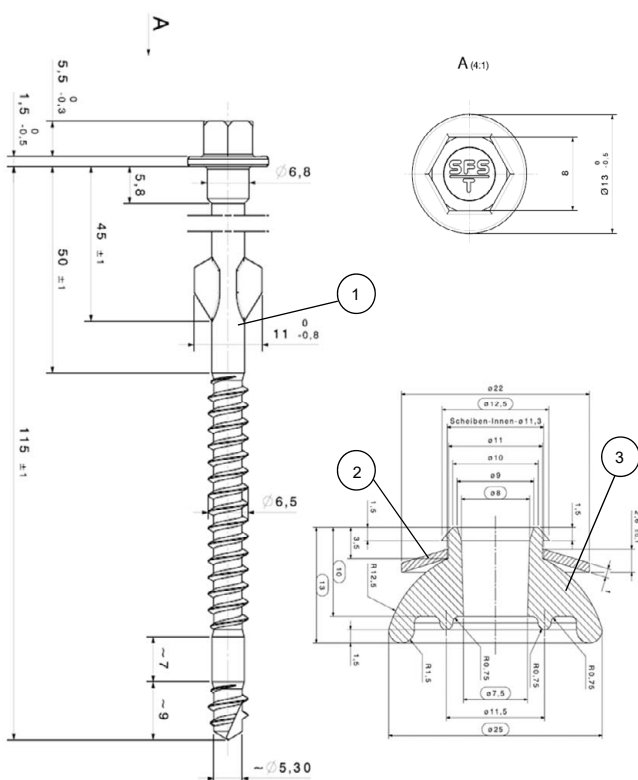
Bild 6: SFS SCFW-C11 6,5 x 115 mm
