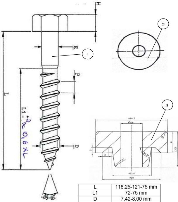
Bild 11: UNI-Bau Vibra-Schraube 1081209 8 x 120 mm
