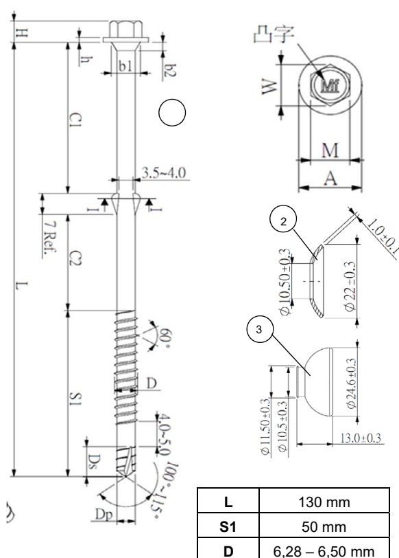
Bild 10: Shen Fung Spezialbohrschraube 6,5 x 130 mm
