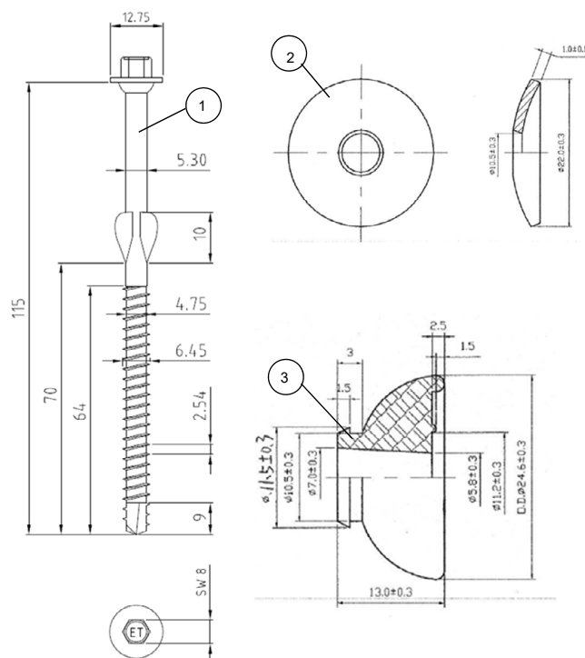
Bild 9: Eurotec 111352 6,5 x 115 mm
