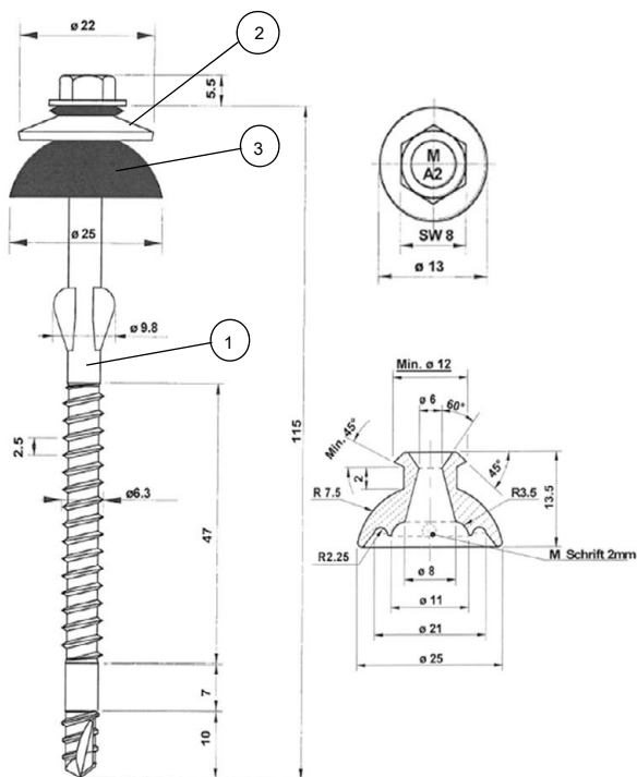
Bild 4: PMJ 745765115E22 6,5 x 115 mm
