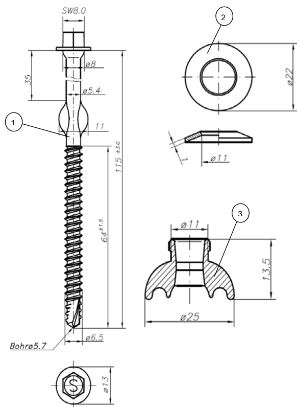
Bild 1: Schmidt SSH 6,5 x 115 mm
