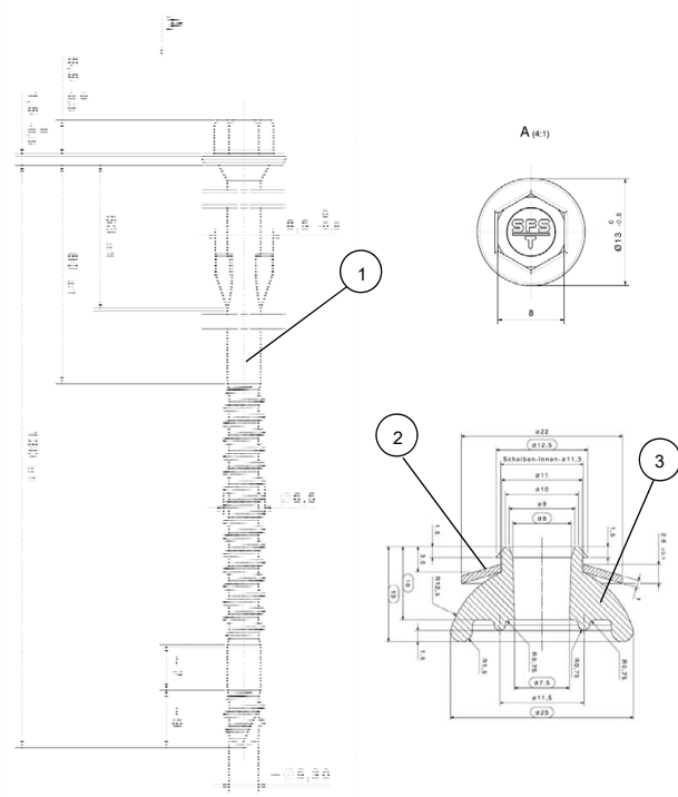
Bild 7: SFS SCFW 6,5 x 130 mm
