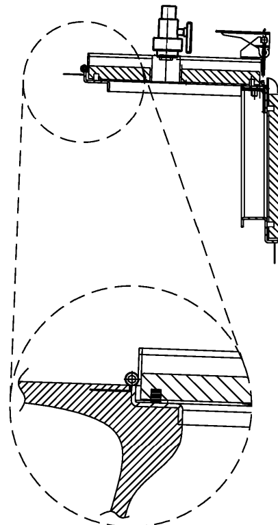
Detail a zeigt Verbindung zwischen GFK und Edelstahlrahmen
