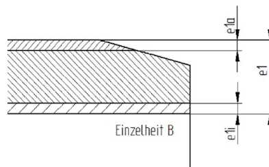
dreischichtiger Rohraufbau gültig im Wanddickenbereich e1
