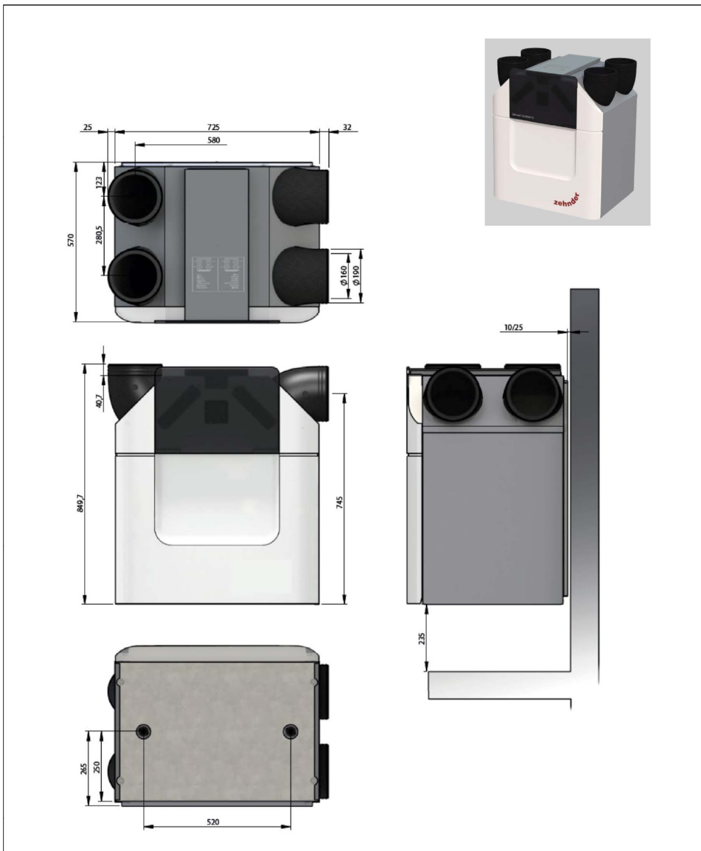
Zentrale Lüftungsgeräte mit Wärmerückgewinnung der Baureihe "ComfoAir Q450"
