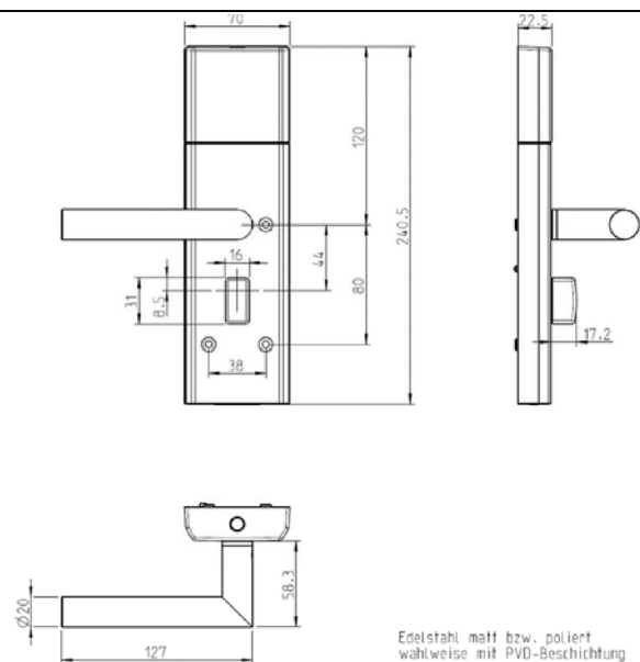
Innenmodul
