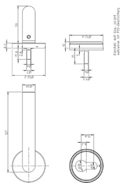
Außenmodul Rosette
