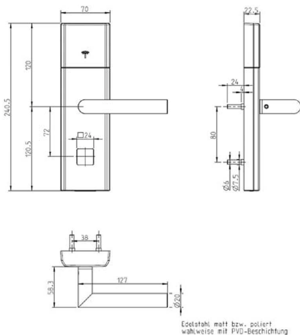
Außenmodul
