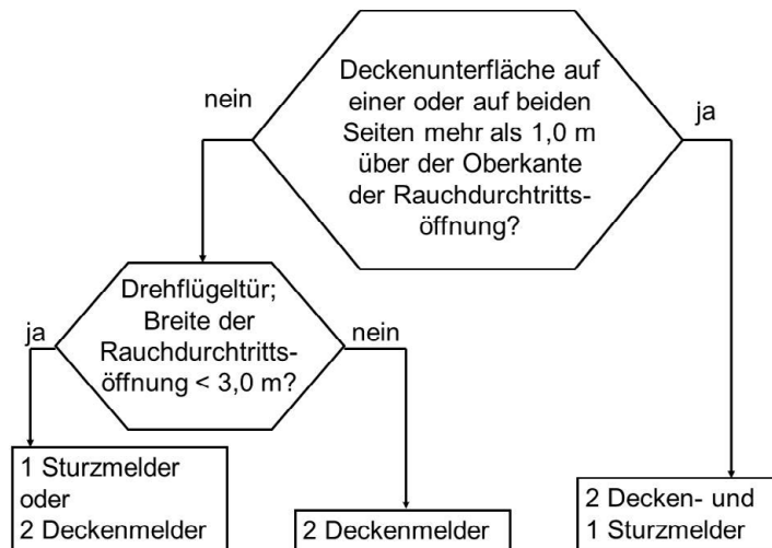
Bild 3: Entscheidungsdiagramm
