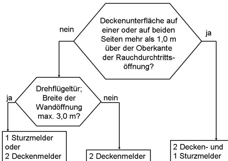
Bild 3: Entscheidungsdiagramm
