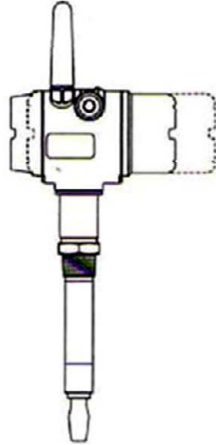
Hygieneanschluss (Standardlänge)
