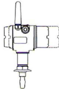
Hygieneanschluss (Standardlänge)
