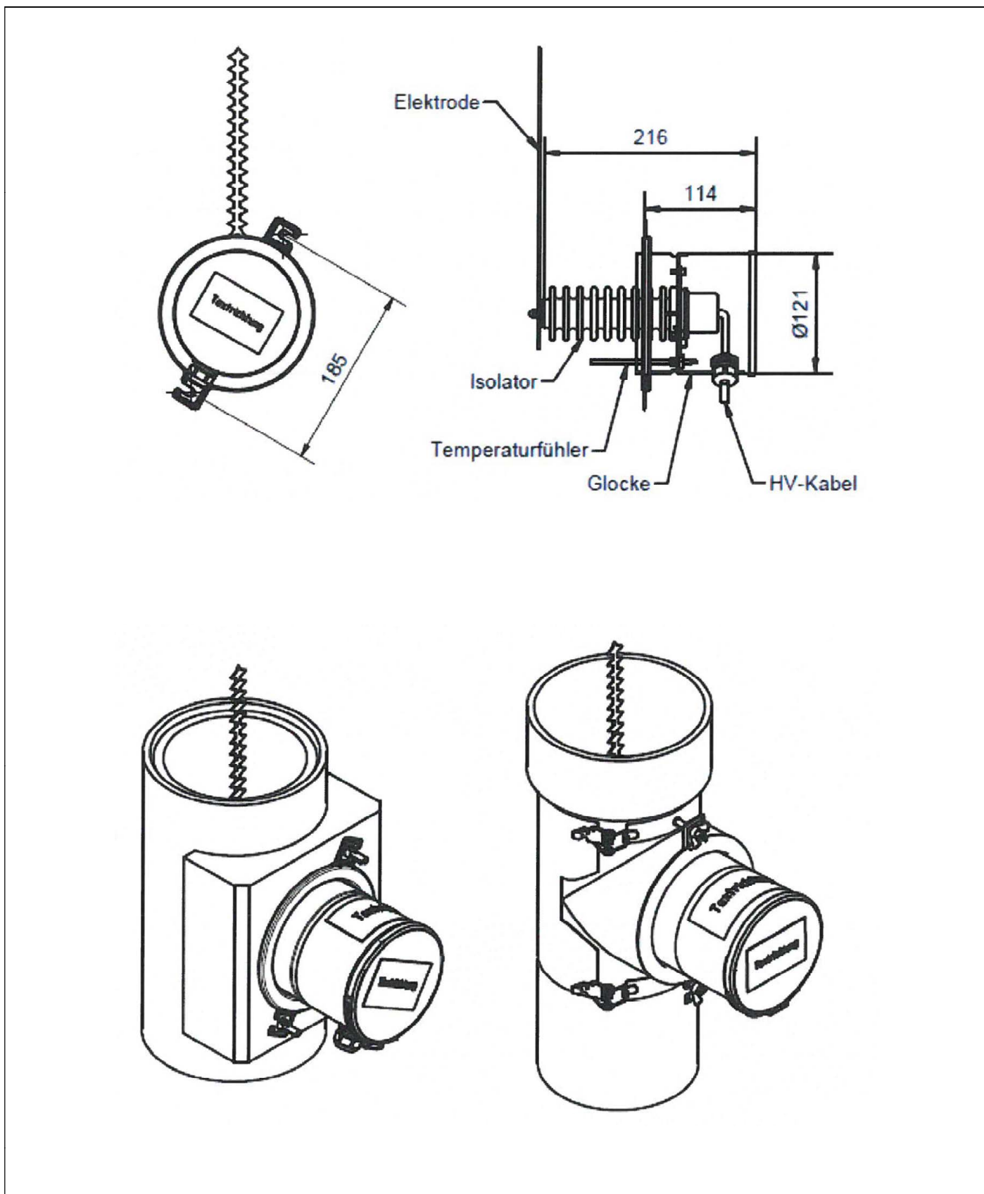
Staubabscheider Typ "Fireclean", "Fireclean 1", "Fireclean 2" "Fireclean 3" und "Fireclean4" für Abgasanlagen
