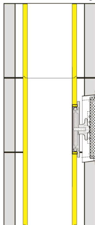
Abgasanlage ohne Wärmedämmung
