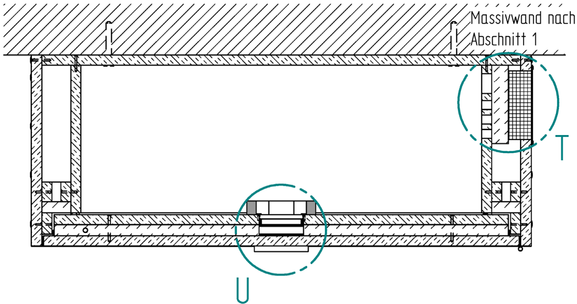
Schnitt H-H
