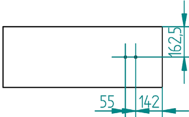
AVENAR-panel 8000 in LS 30, Rückwand Ansicht LS 30 Decke Innen Befestigung Rauchmelder
