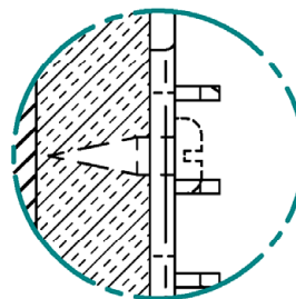
Detail Y Befestigung AVENAR-panel Rückwand
