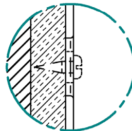
Detail Z Befestigung AVENAR-panel Rückwand
