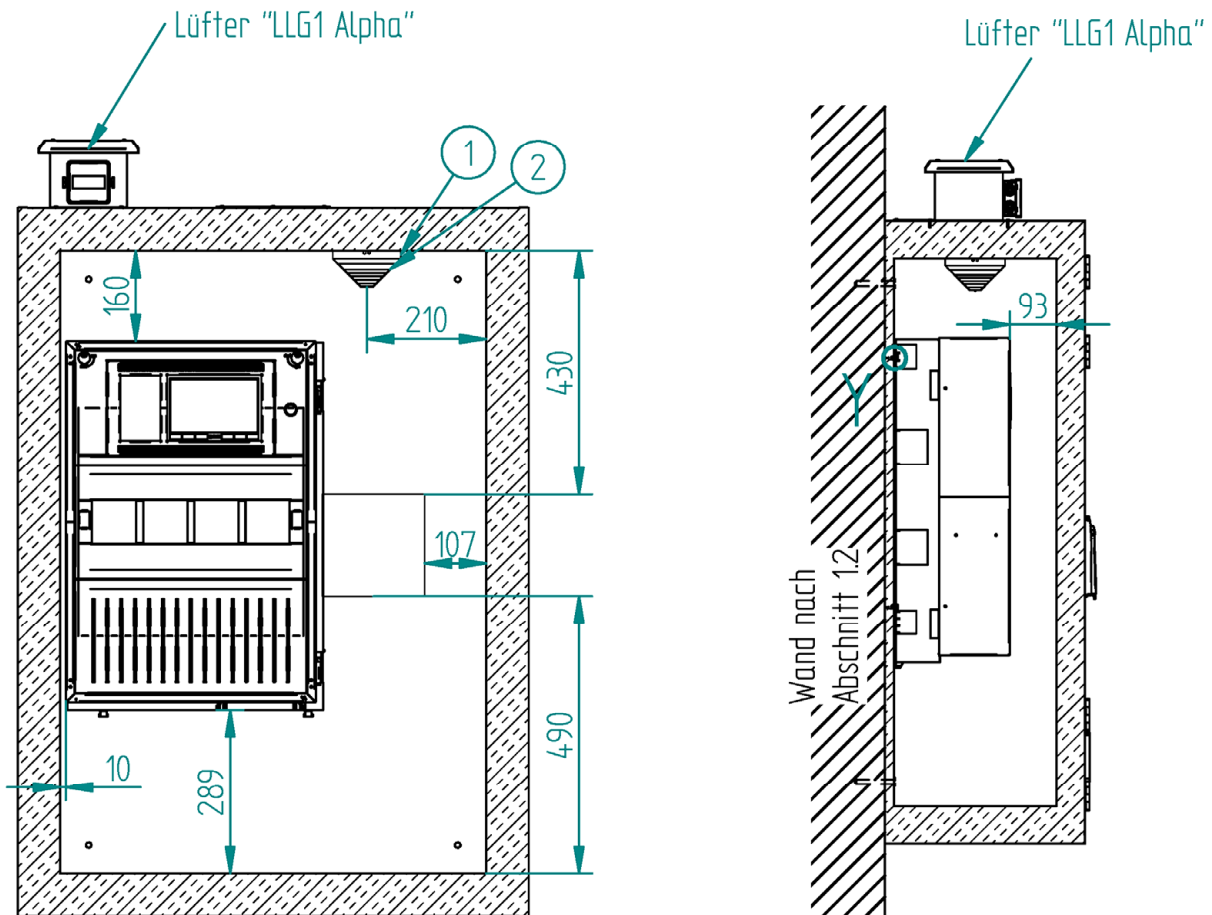
Detail Y Befestigung AVENAR-panel Rückwand
