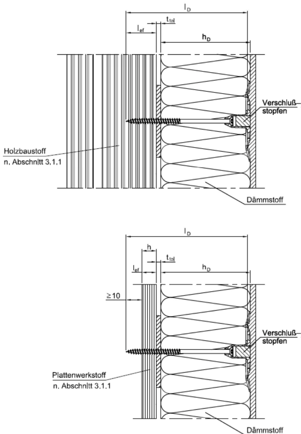
Einbausituation ejotherm STR H und ejotherm STR H E mit Zusatzsteller VT 90, oberflächenbündige Dübelmontage
