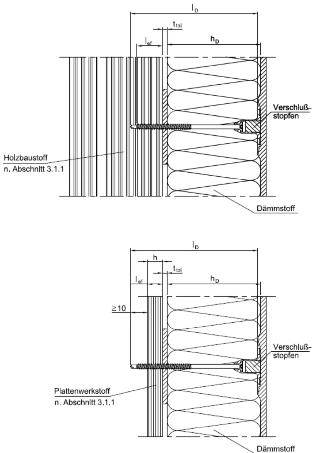
Einbausituation ejotherm STR H A2, oberflächenbündige Dübelmontage
