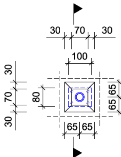
Draufsicht
