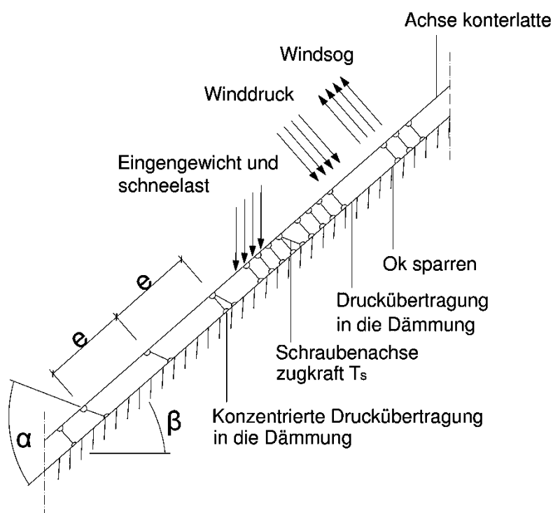
Abbildung A.4.1: Befestigung von Aufdach-Dämmsystemen auf Sparren- Statisches Modell für parallel angeordnete Schrauben
