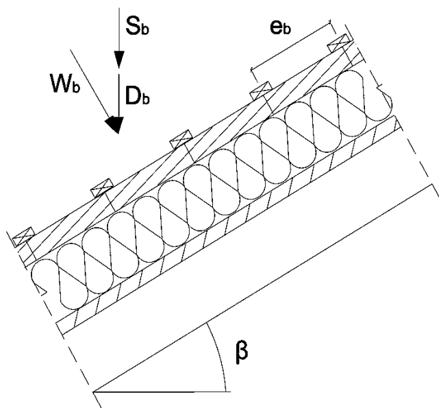
Abbildung A.4.2: Einzellasten F_b rechtwinklig zu den Konterlatten
