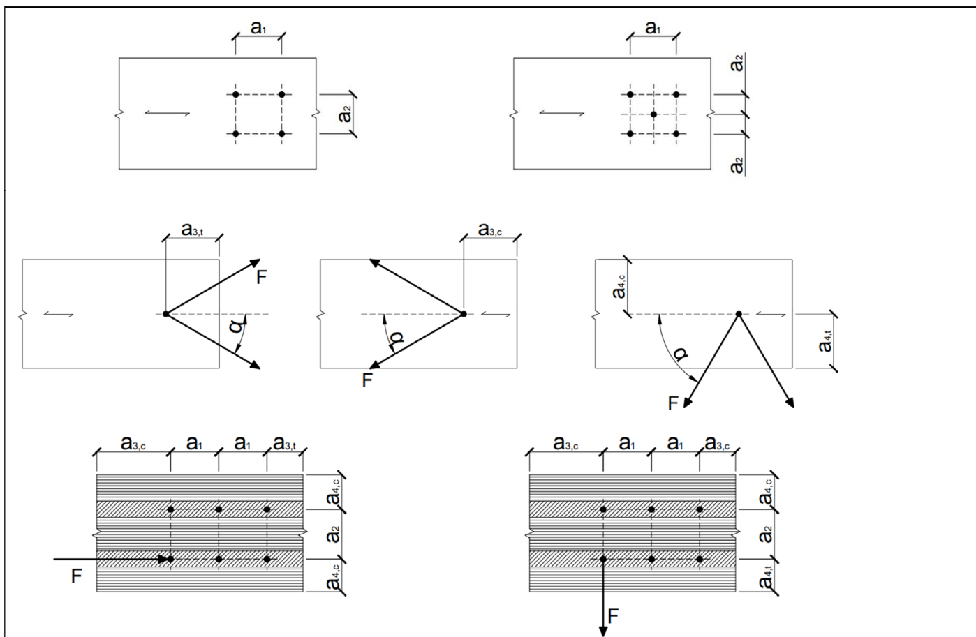
Abbildung A.2.2 Definition der Mindestabstände in den Schmalflächen des Brettspertholzes. Bei Schrauben in den Schmalflächen sind die Abstände a_1 und a_3 parallel zur Seitenfläche sowie die Abstände a_2 und a_4 rechtwinklig zur Seitenfläche des Brettspertholzes
