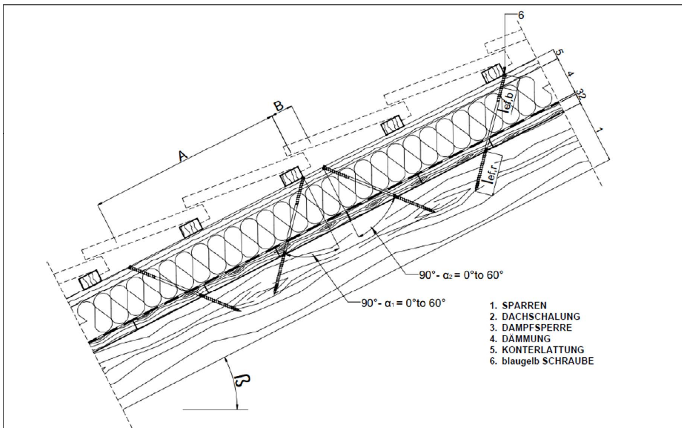
Abbildung A.6.4 Befestigung der Aufdach-Dämmung auf Sparren – Prinzipdarstellung mit wechselnder Neigung angeordneter Schrauben
