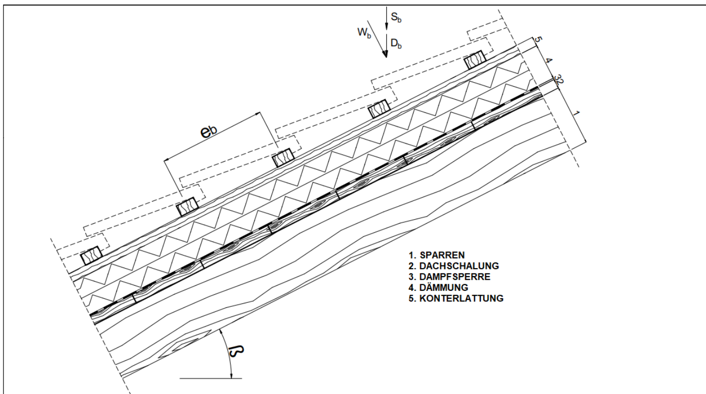
Abbildung A.6.2 Einzellasten F_b rechtwinklig zu den Konterlatten
