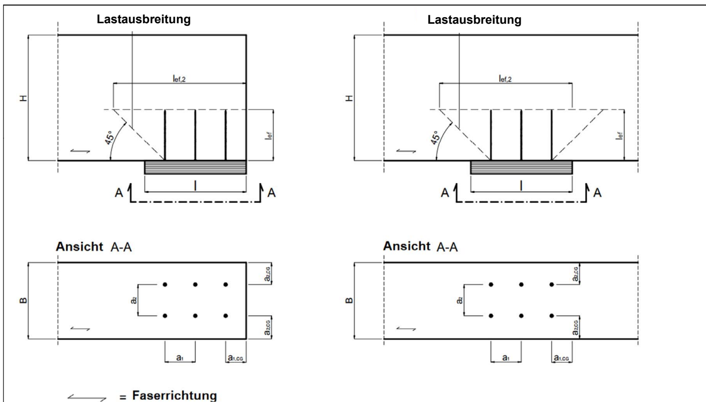
Abbildung A.3.1 Verstärktes Endauflager (links) und verstärktes Zwischenaflager (rechts)
