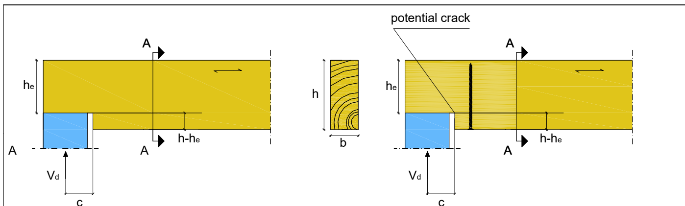
Abbildung A.4.2 Beispiel für die Verstärkung einer Ausklinkung bei Zugbeanspruchung rechtwinklig zur Faser
