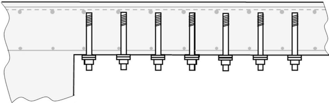
Einbauzustand
