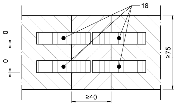
Schnitt A-A
