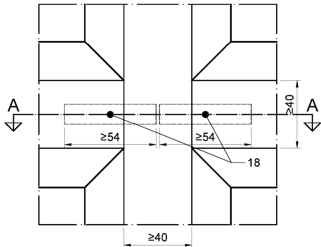
Dübel-Verbindung
