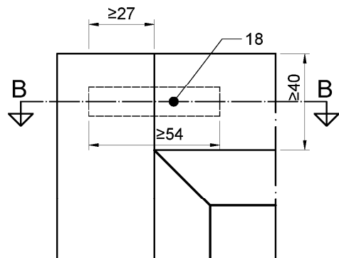
Dübel-Verbindung
