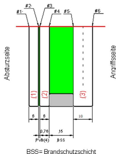
Abb.1: Scheibenaufbau von "Promat-SYSTEMGLAS F1-30"
