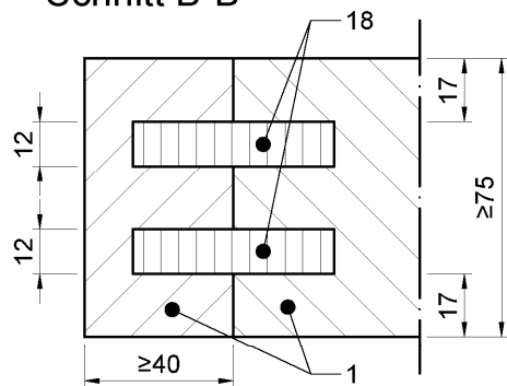
Schnitt B-B
