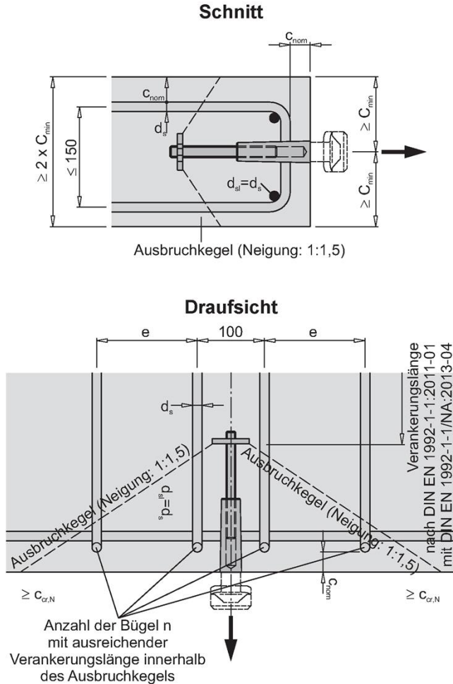
Bild 23: Einbausituation Stirnseite - Zugbeanspruchung mit Rückhängebewehrung - Bewehrungslage
