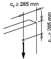
Bild 20: Einbausituation Wandfläche - Querbeanspruchung ohne Betonkantenbruch, ohne Rückhängebewehrung für Aufhängekonus 15,0 für Isolierungen bis 11cm
