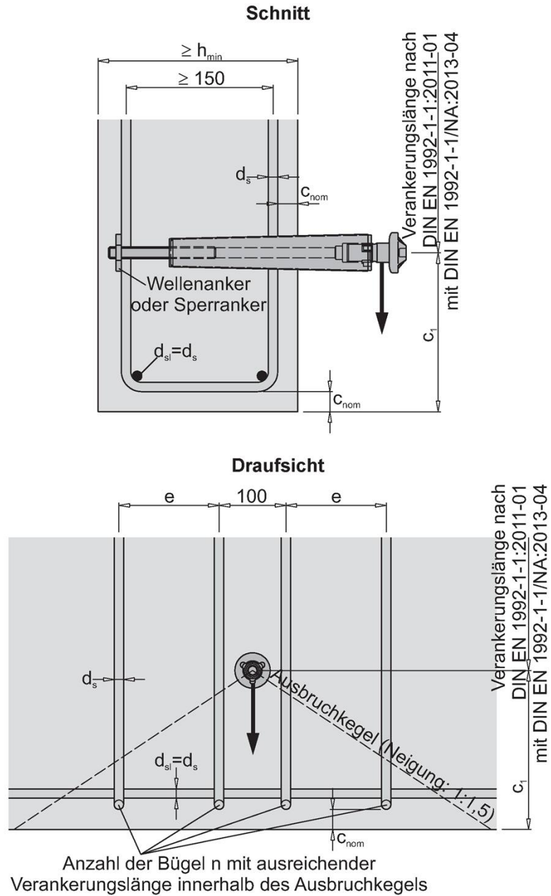
Bild 28: Einbausituation in Wänden - Querbeanspruchung mit Rückhängebewehrung - Bewehrungslage
