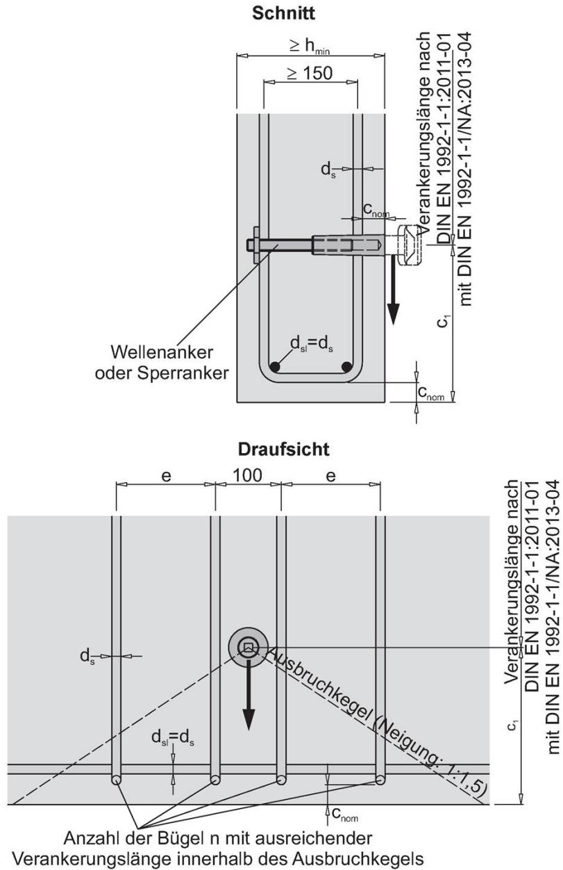
Bild 27: Einbausituation in Wänden - Querbeanspruchung mit Rückhängebewehrung - Bewehrungslage
