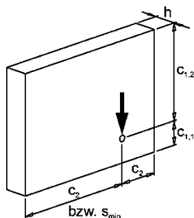
Bild 21: Randabstände bei Querbeanspruchung
