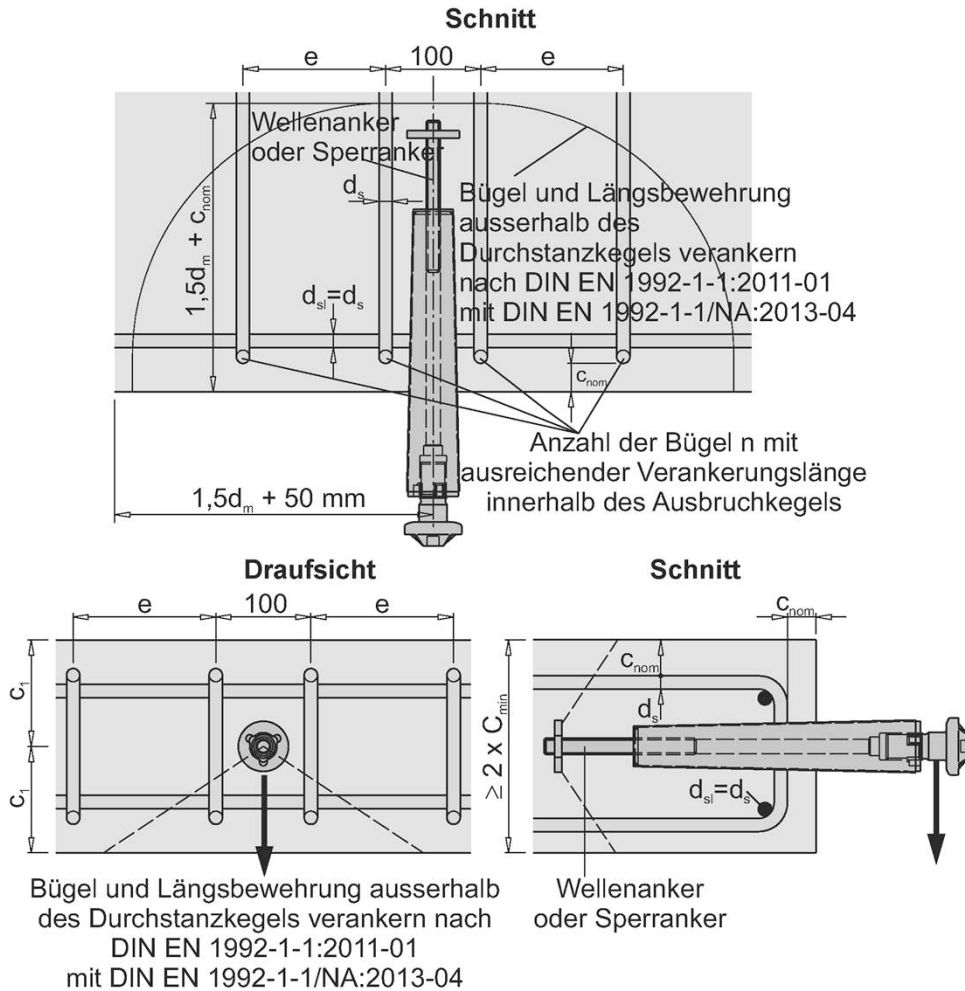
Bild 30: Einbausituation Stirnseite - Querbeanspruchung mit Rückhängebewehrung - Bewehrungs- lage
