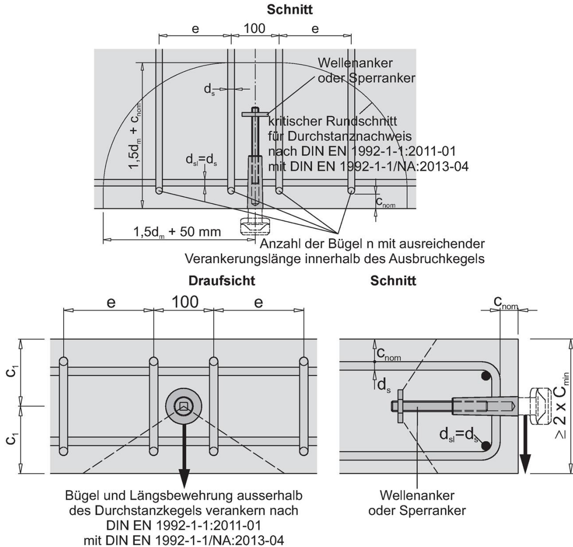
Bild 29: Einbausituation Stirnseite - Querbeanspruchung mit Rückhängebewehrung - Bewehrungslage
