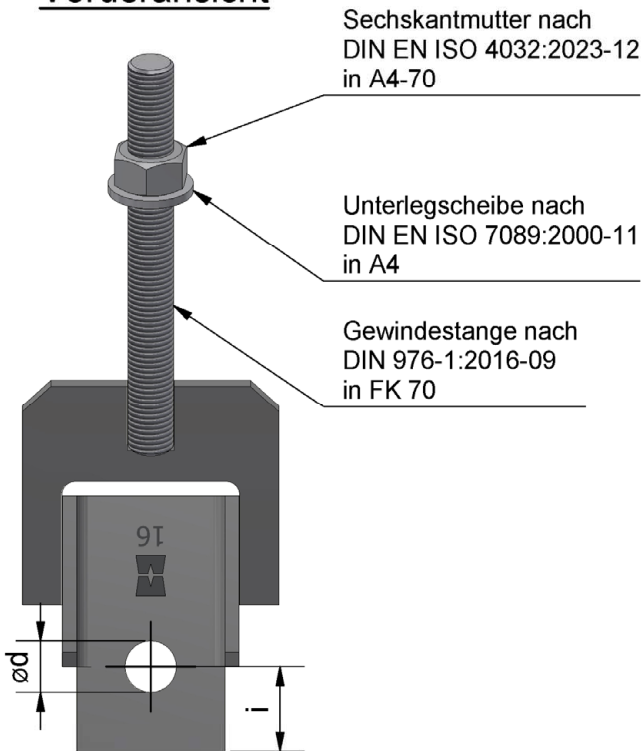
Vorderansicht
