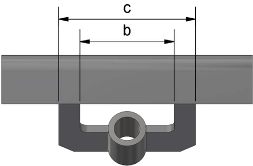
Draufsicht
