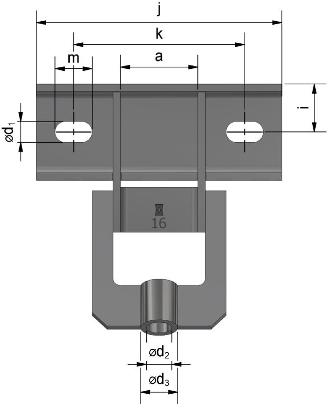
Vorderansicht
