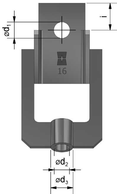
Draufsicht
