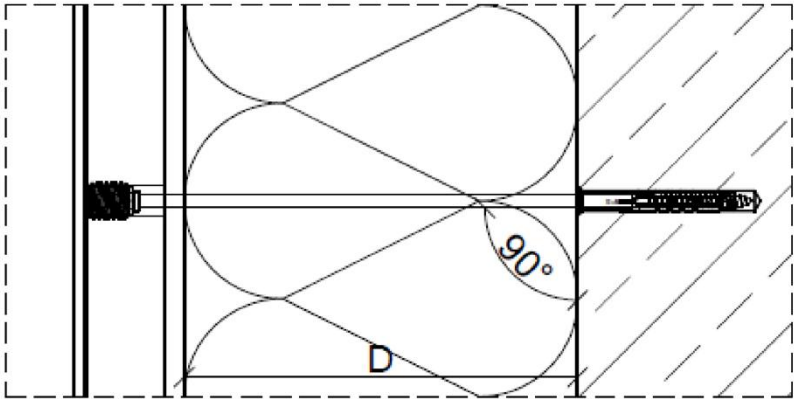
Detail horizontale Verschraubung (Ansicht)
