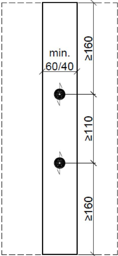
Detail horizontale Verschraubung (Ansicht)
