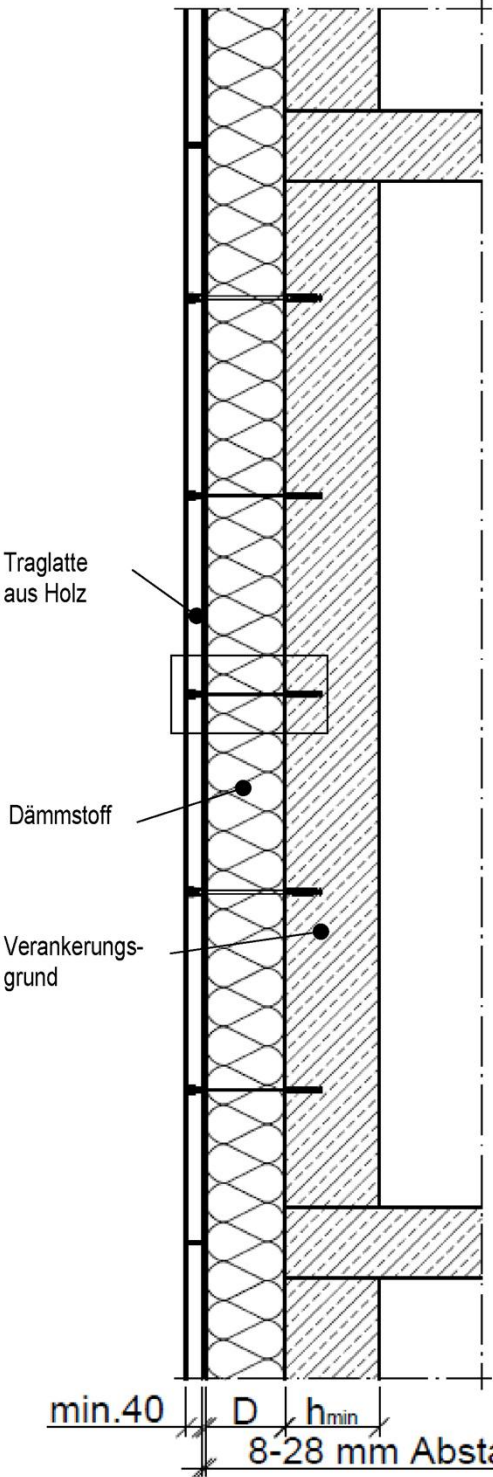
Detail horizontale Verschraubung (Ansicht)
