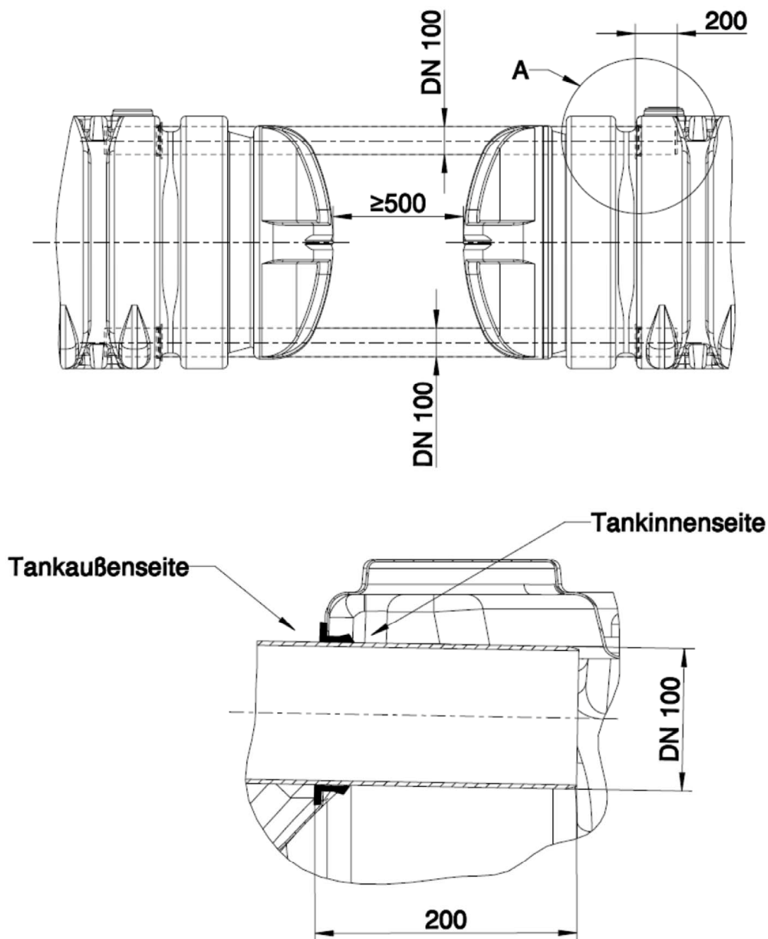
Detail Dichtung montiert mit Rohr
