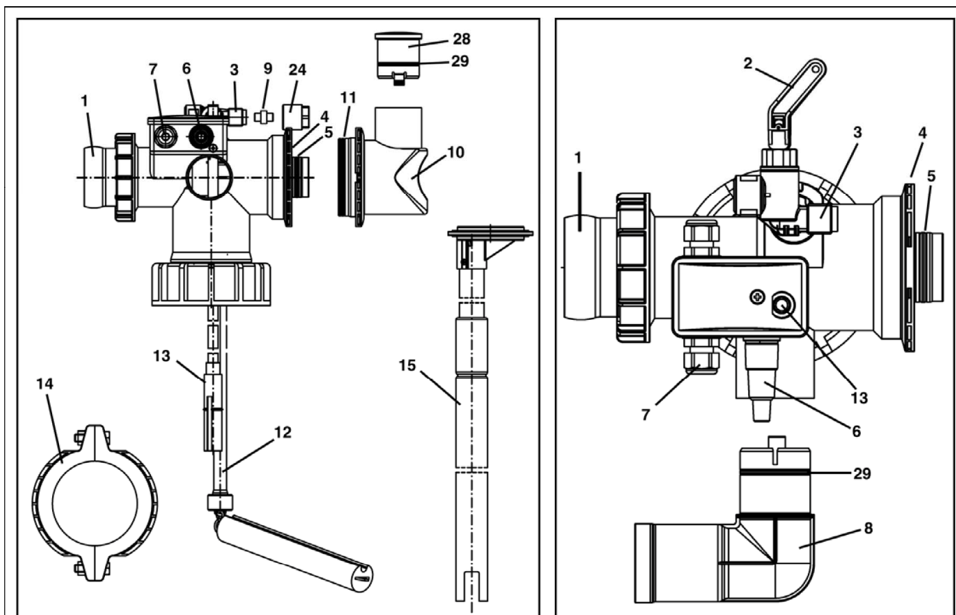
Bild 1: Grundeinheit mit Zubehör
