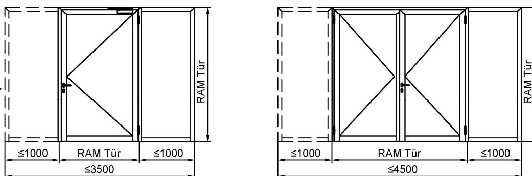
T30-1-(RS)-Tür T30-2-(RS)-Tür -mit Seitenteil(en)-
