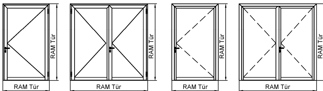
T30-1-(RS)-Tür T30-2-(RS)-Tür -Grundvarianten-
