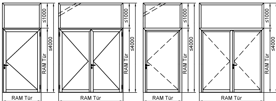
T30-1-(RS)-Tür T30-2-(RS)-Tür -mit Oberteil-
